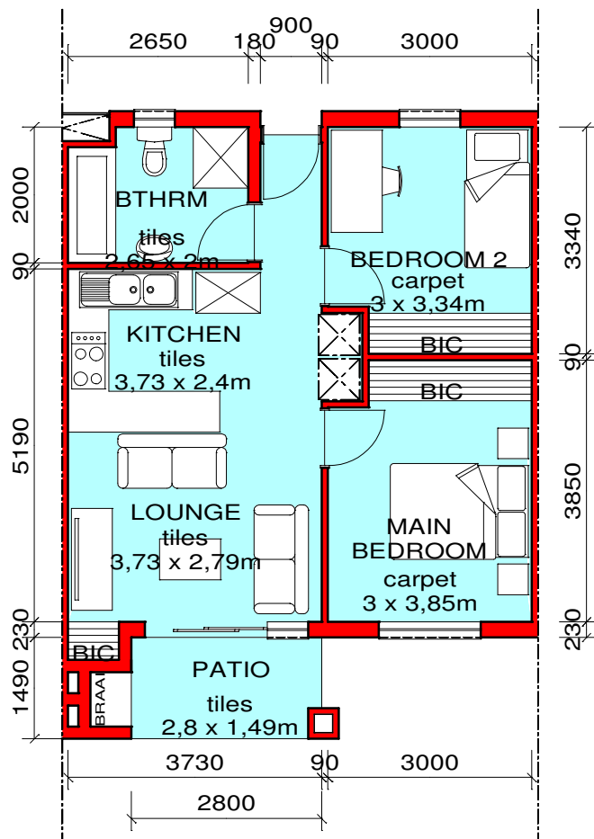
UNIT TYPE B 2 BEDROOM UNIT 59.84 SQ/M (INCL. 4,17 SQ/M BALCONY & BRAAI)
