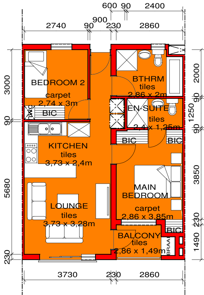
UNIT TYPE A 2 BEDROOM UNIT 116,4 SQ/M (INCL. 4,26 SQ/M BALCONY & BRAAI)
